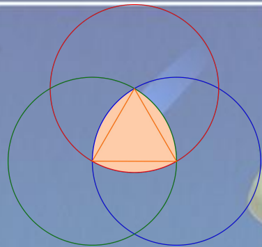
勒洛三角形 Reuleaux triangle
